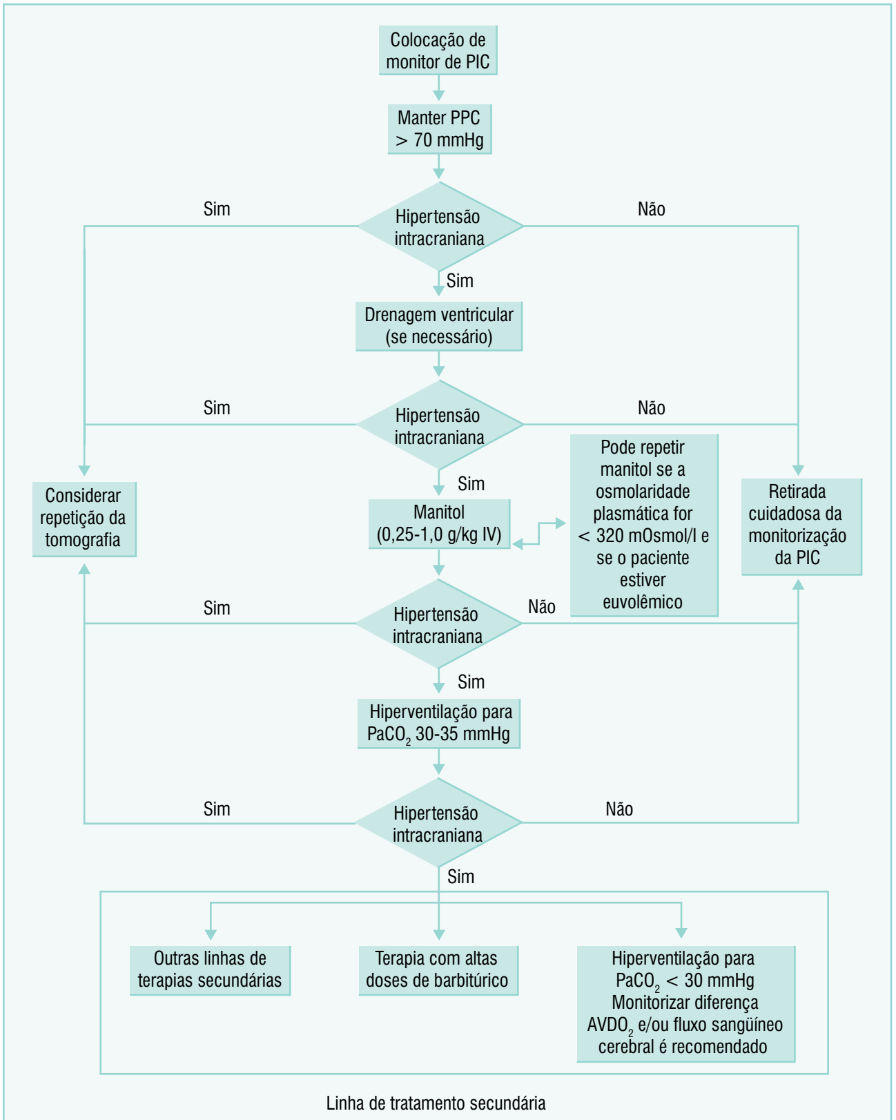
FIGURA 10 – Algoritmo para tratamento de hipertensão intracraniana no TCE grave.
